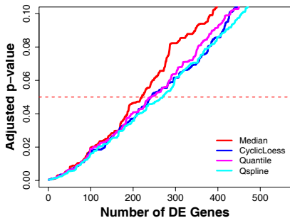
T-test
