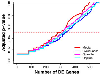
T-test (perm)
