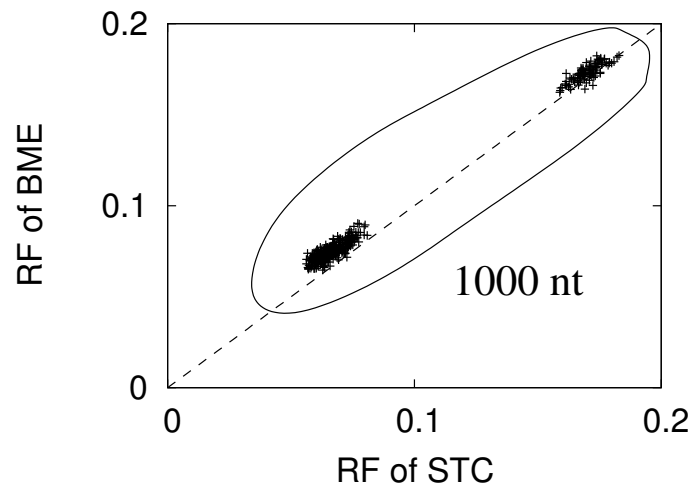
(d) STC versus BME (5000 taxa)
