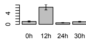
GgaAffx.8887.1.S1_s_at (RCJMB04_35G11)
