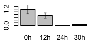
GgaAffx.11653.1.S1_s_at (RCJMB04_3F1)
