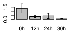
GgaAffx.5963.1.S1_at (RCJMB04_7N4)
