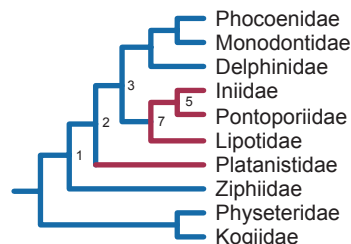
R) Yan et al. 2005 Bayes, P: mt genome (AAs)
