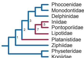
T) May-Collado and Agnarsson 2006 Bayes: 1 mt gene
