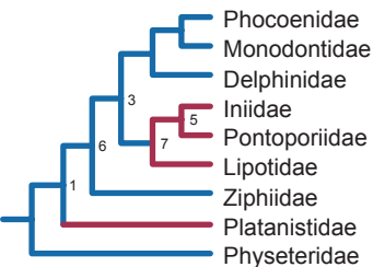
P) Nikaido et al. 2001 ML: 12 nu genes
