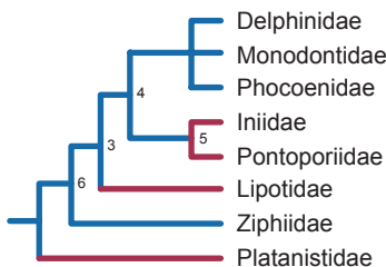
Q) Yang et al. 2002 ML, P, NJ: 1 mt gene
