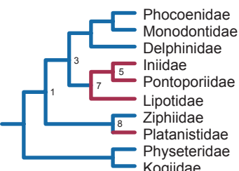
Y) Yang 2009 Bayes: mt genome
