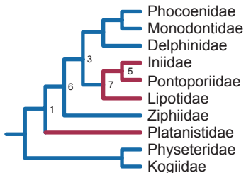
W) Steeman et al. 2009 Bayes: 9 nu+6 mt genes
