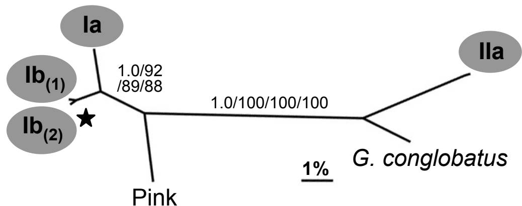
(B) G. ruber/ G. conglobatus
