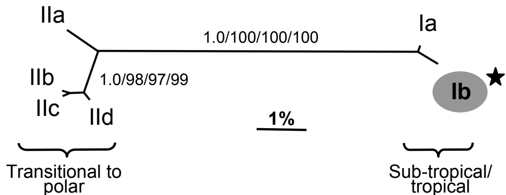
(D) T. quinqueloba
