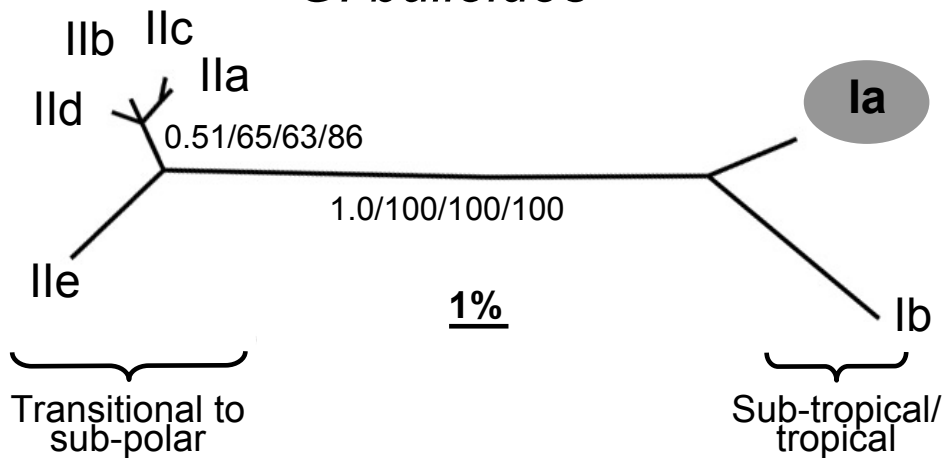
(C) G. bulloides
