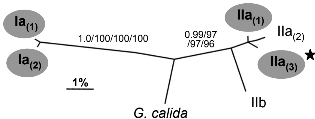
(A) G. siphonifera/ G. calida
