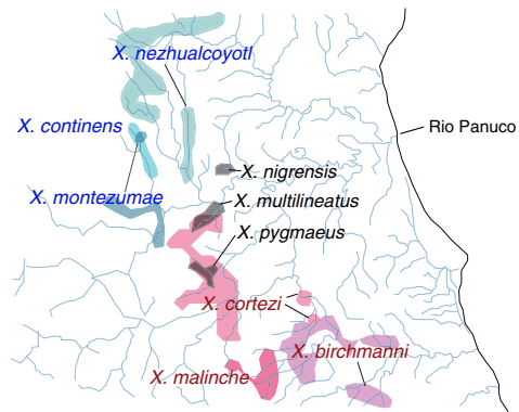
(d) geographical distributions of the northern swordtails
