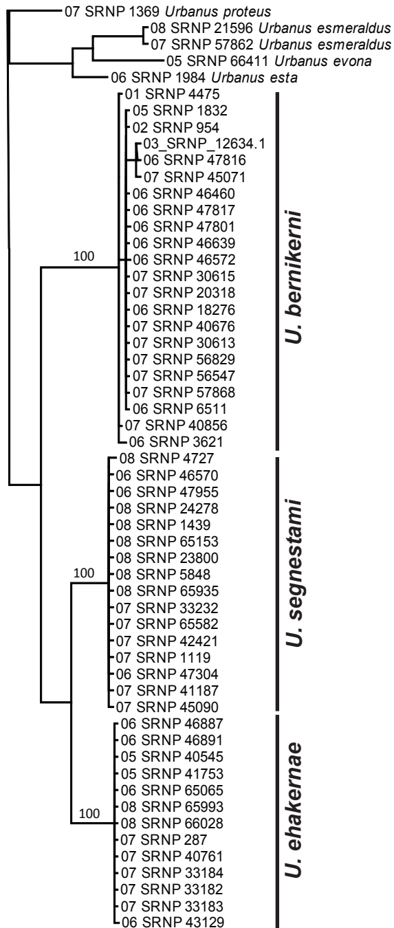
(a) COI
