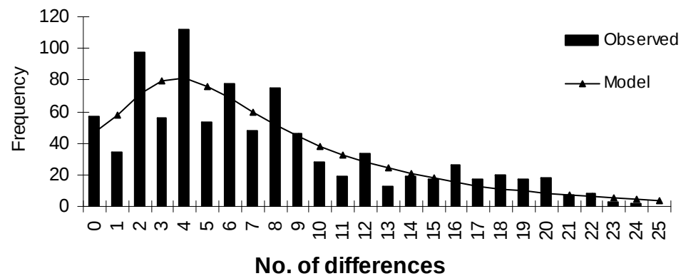
Mismatch Distribution ( G. g. domesticus )
