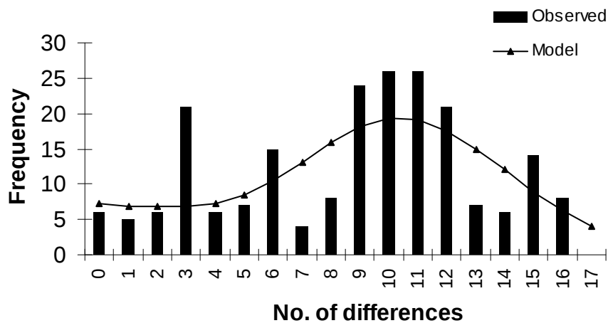
Mismatch Distribution ( G. g. gallus )
