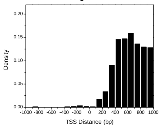
M.grisea
