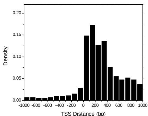
S.cerevisiae
