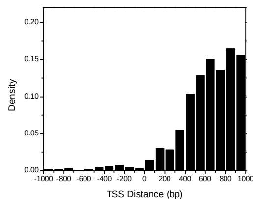
N.crassa
