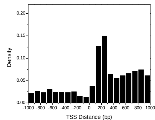
O.sativa
