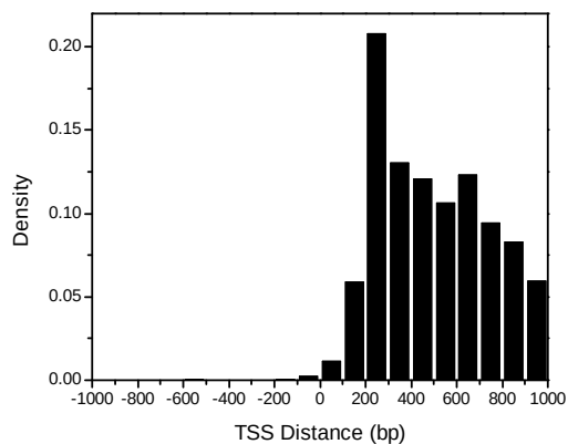
M.grisea
