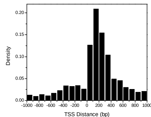
A. mellifera
