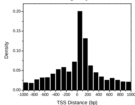
G.gallus
