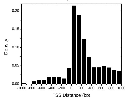
E.gossypii
