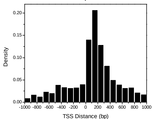
C.familiaris
