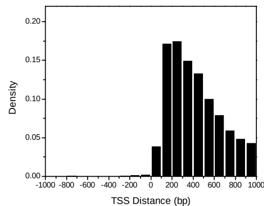
N.crassa
