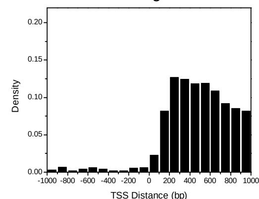
S.pombe
