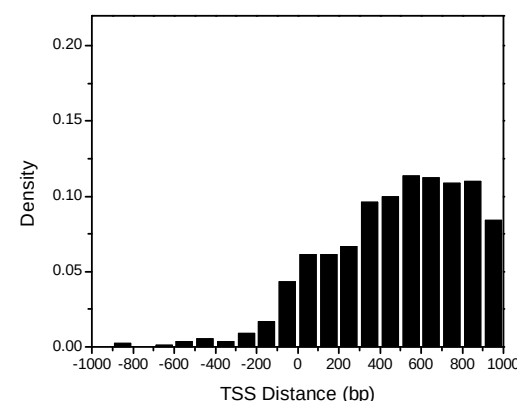
K.lactis
