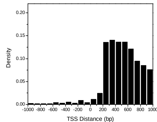
A.thaliana
