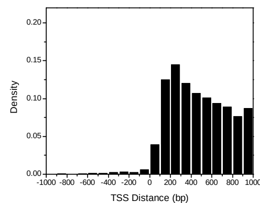
A.thaliana
