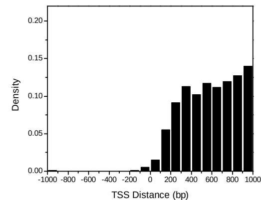
O.sativa
