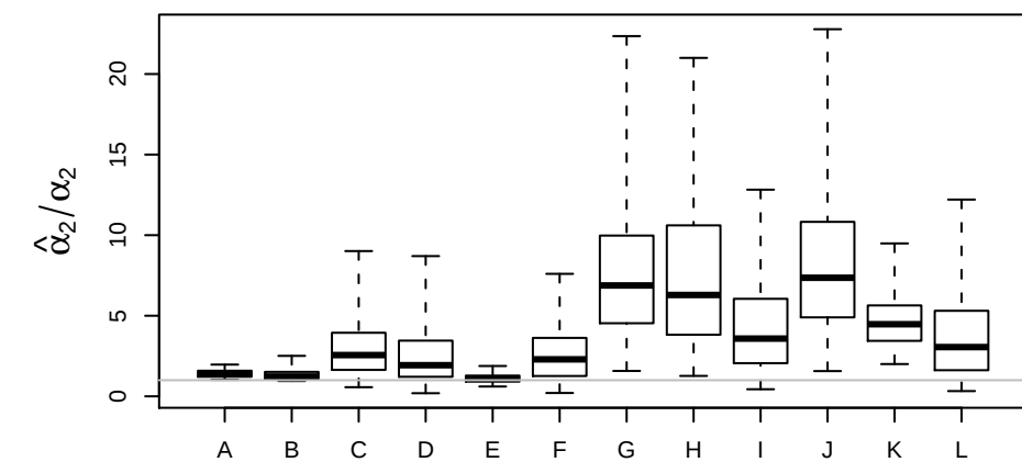
Data set
