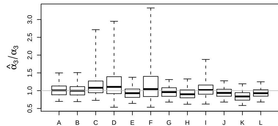
Data set
