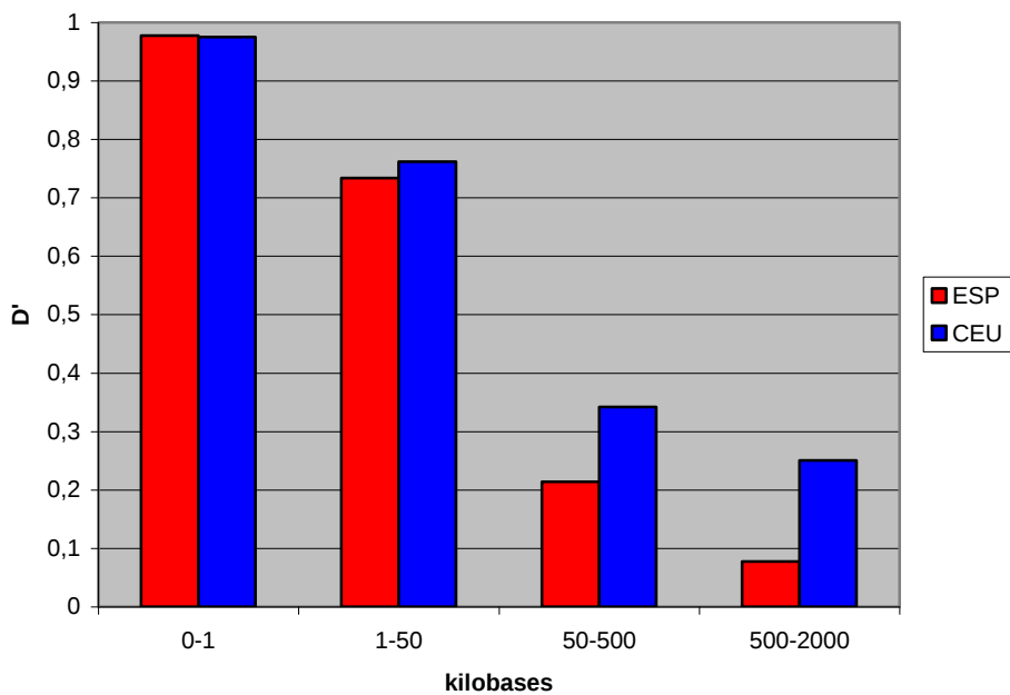
LD Decay ( D' )
