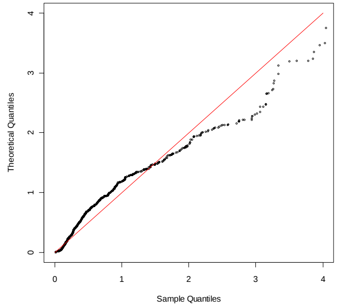
QQ-plot distr. Gamma. Chr-7
