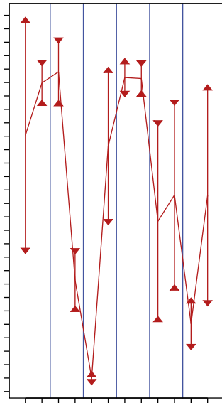
(D) Ckm
