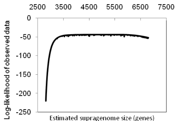
Haemophilus influenzae (13 strains) [ supragenome estimate 5170 genes ]
