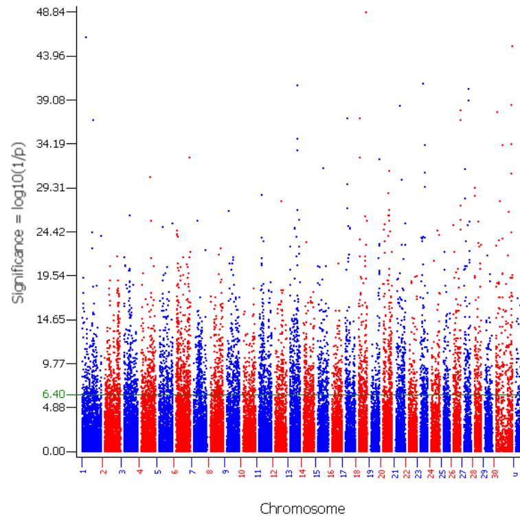
Manhattan Plot: PY
