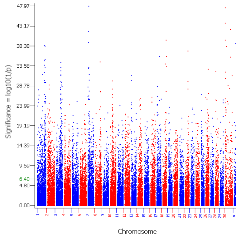
Manhattan Plot: DPR
