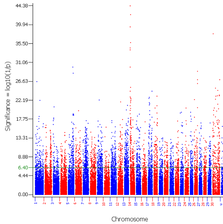
Manhattan Plot: FPC
