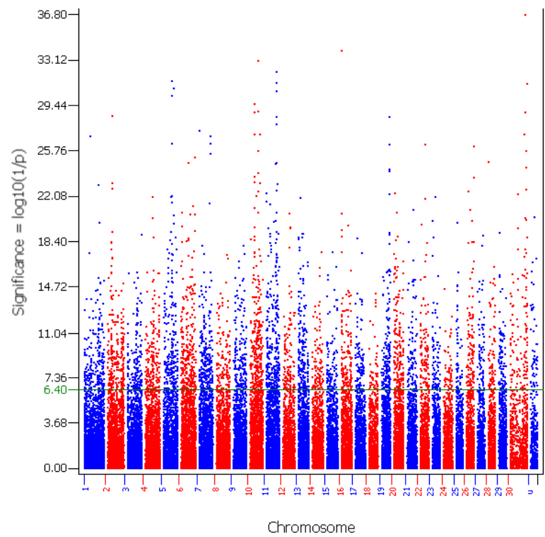
Manhattan Plot: FS
