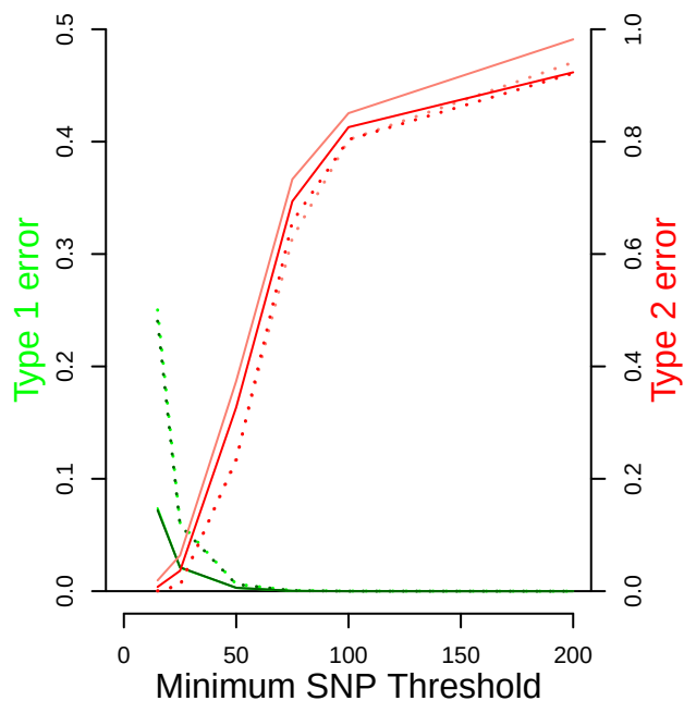
PLINK – modpruned SNP data
