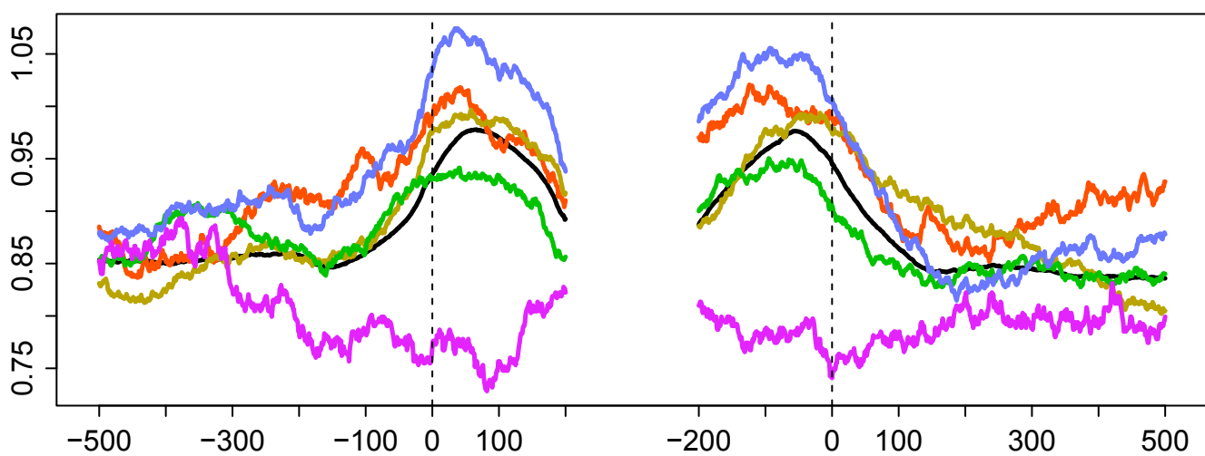
Input_GM12878
