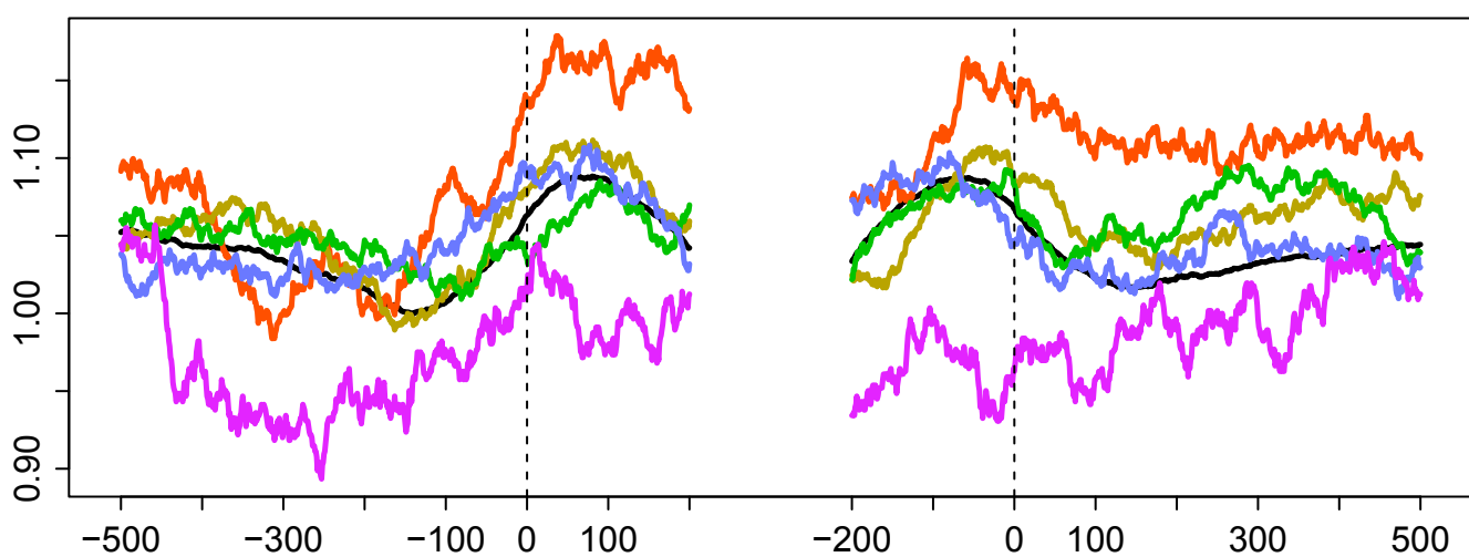
Input_K562
