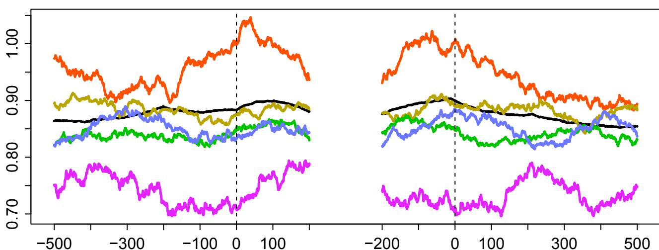
Input_Hep G2
