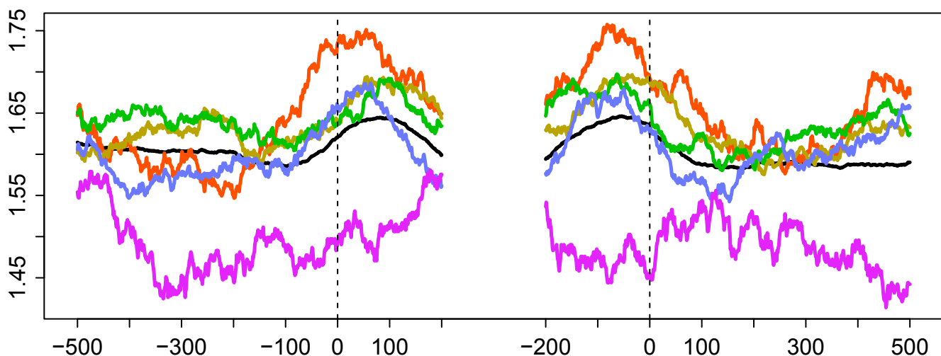
Input_H1 hESC
