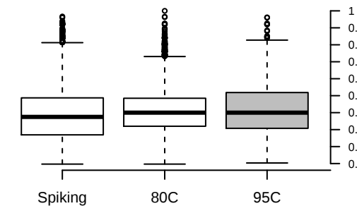
Spiking
