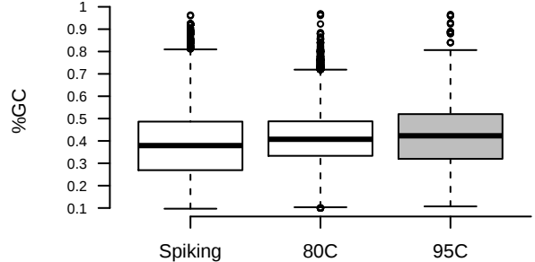
Spiking
