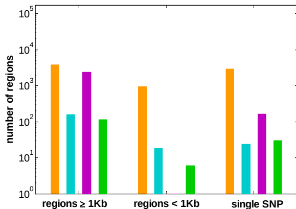
PCA merge - CNPs
