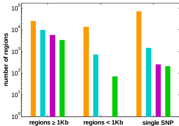
PCA merge - CNVRs
