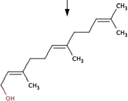
Farnesol
