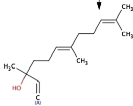
Nerolidol
