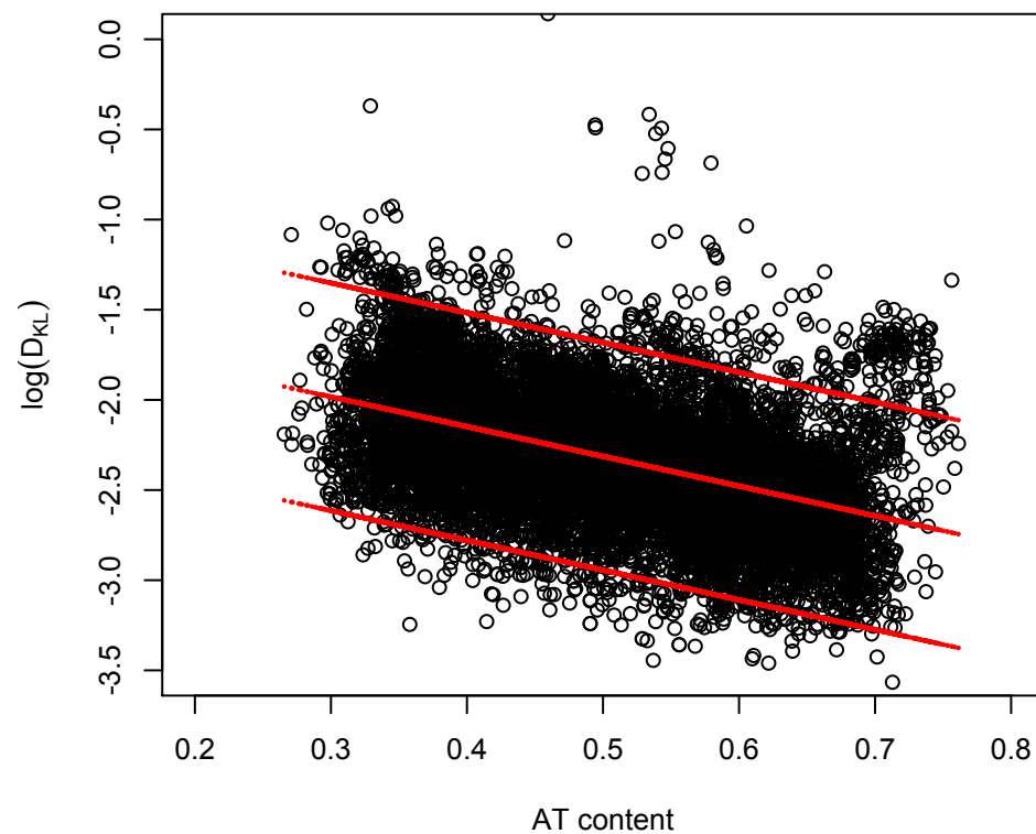
GIs
