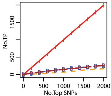
(b) Scenario 1: dataset 11
