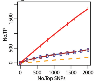
(g) Scenario 2: dataset 21
