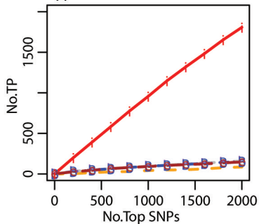
(f) Scenario 2: dataset 11
