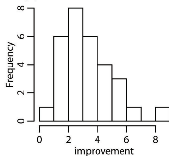
(d) Scenario 1: dAUC Hist.
