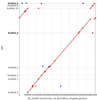
Ion + 110X PacBio
