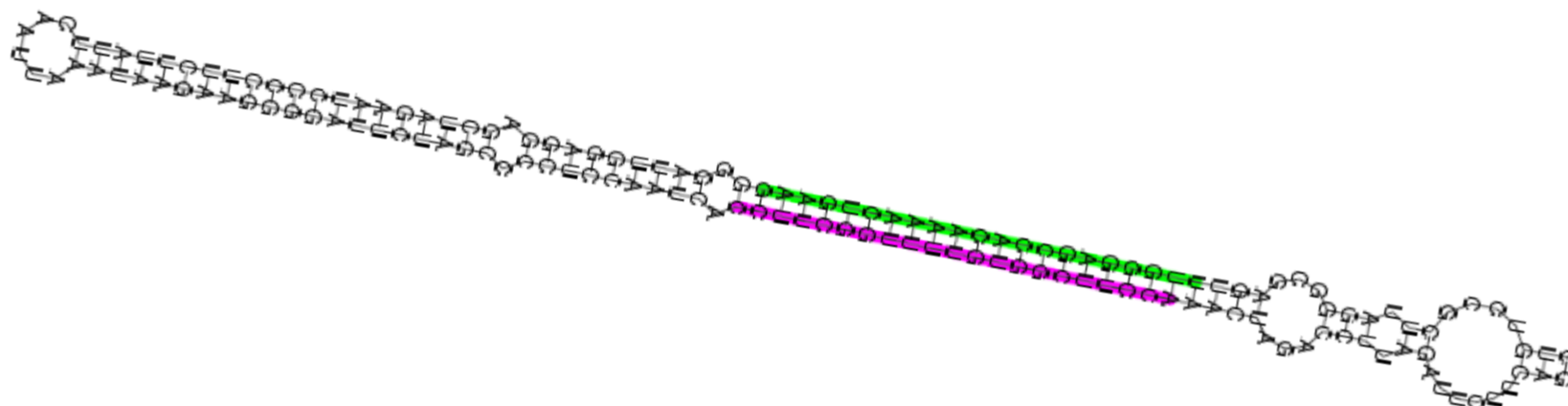
Zma_miR_Seq15_chromosome5 _ 167348311_167348332
