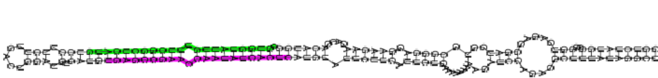
Zma_miR_Seq09a_chromosome10 _137316440_137316461
