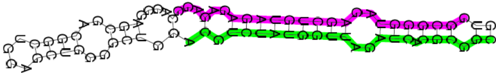
Zma_miR_Seq05_chromosome4_ 19368136_19368159
