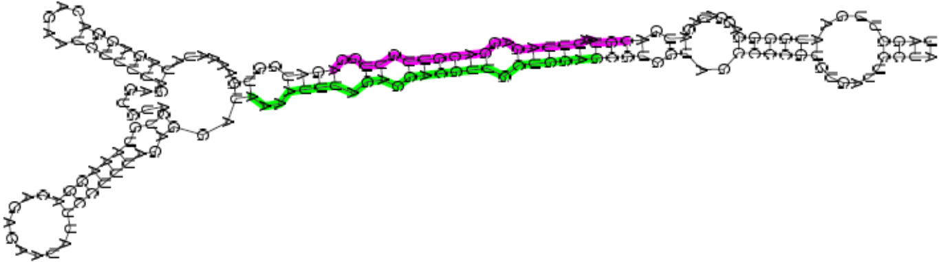
Zma_miR_Seq02_chromosome2 _ 137641787_137641810
