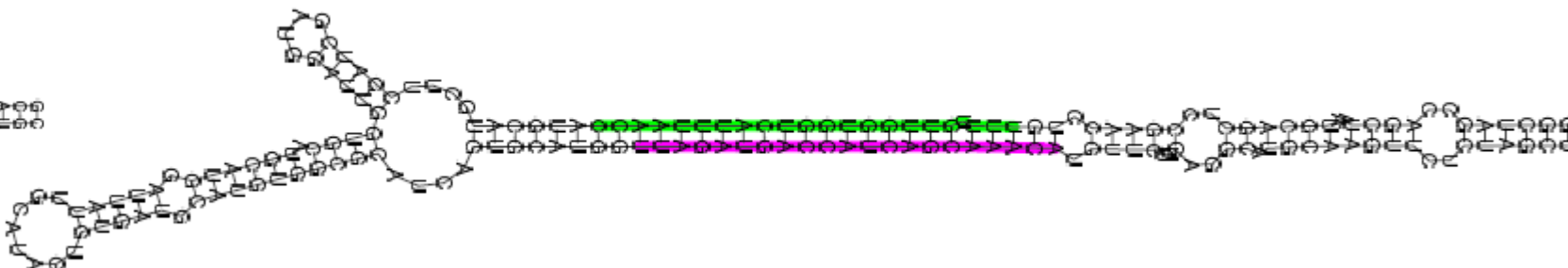
Zma_miR_Seq15_chromosome5 _ 167348311_167348332
