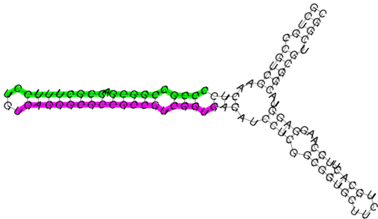
Zma_miR_Seq07b_chromosome1_116745346_116745366
