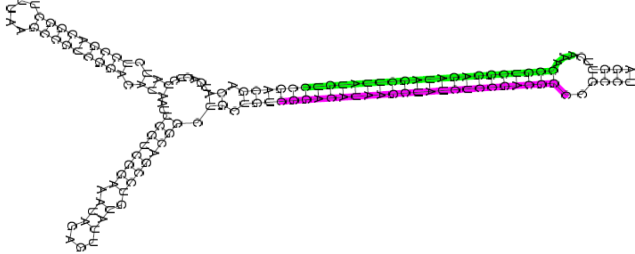
Zma_miR_Seq03_chromosome1 _ 203890843_203890866
