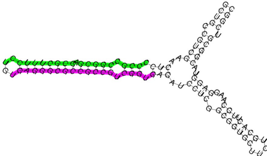
Zma_miR_Seq08_chromosome2_169527754_169527774
