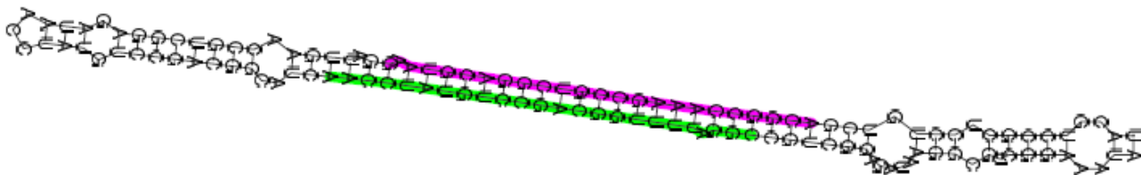
Zma_miR_Seq03_chromosome1 _ 203890843_203890866
