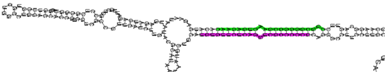
Zma_miR_Seq08_chromosome2_169527754_169527774
