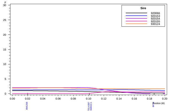
Haley-Knott QTL Analysis: Chromosome 20 DAG1
