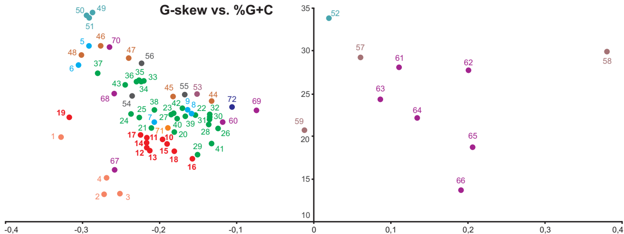
G-skew vs. %G+C
