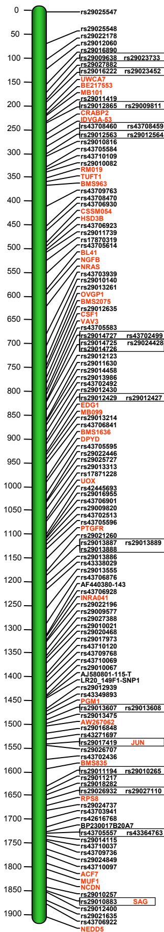
BBU6 – new RH map
