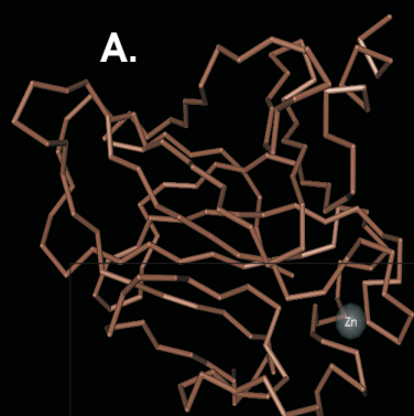
p53
