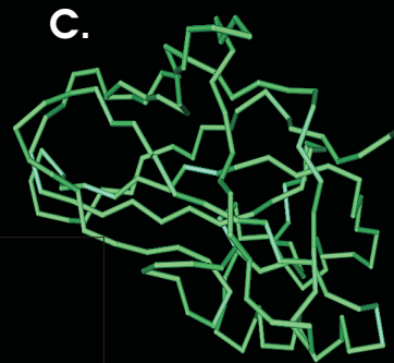
p65
