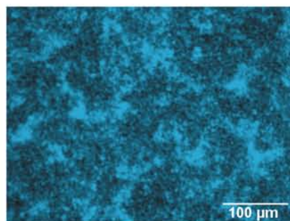
Rt2472(pRC24)
