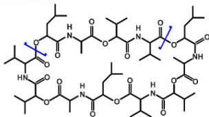
Cereulide
