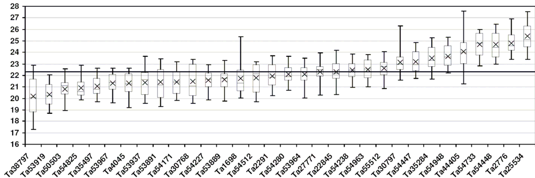
Ct values
