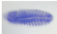
(h) Df31
