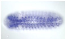
(j) dUTPase
