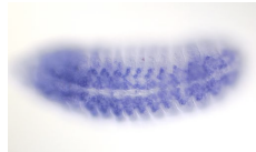
(d) fzy
