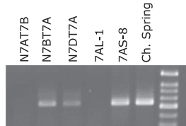
TaHKT2;1 7AL-1
