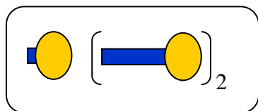
Ceratopteris richardii
