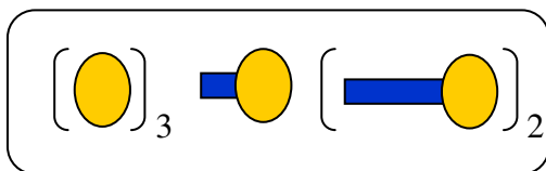
Lactuca serriola
