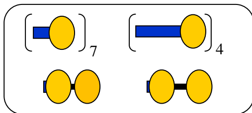
Picea sitchensis
