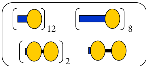
Pinus taeda
