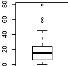
anisoptera
