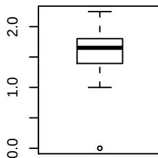
box-cox(anisoptera)
