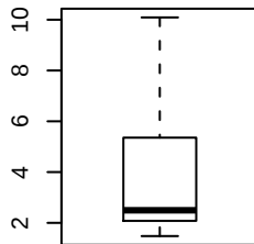
width
