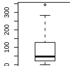
ephemeroptera
