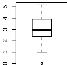
box-cox(ephemeroptera)
