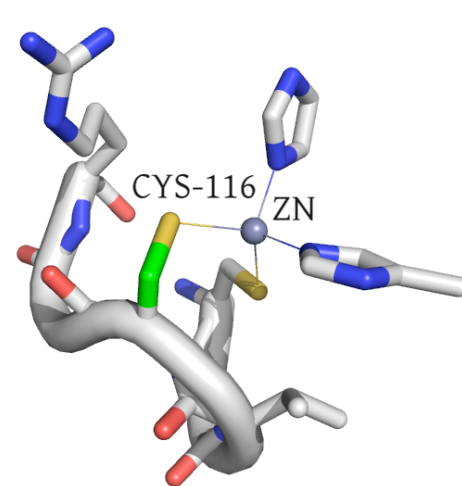
2DRP:A
