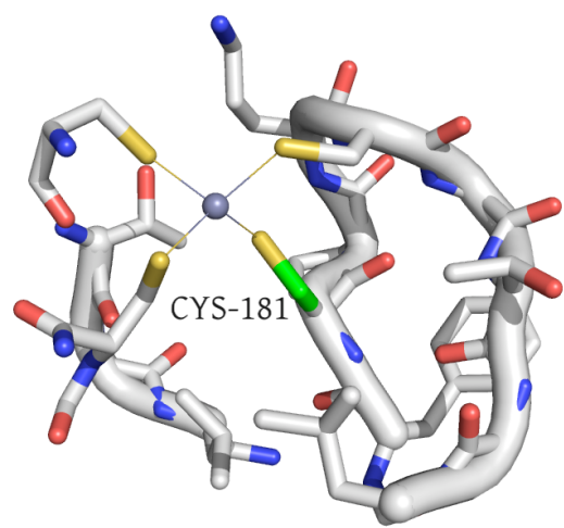
1JZQ:A
