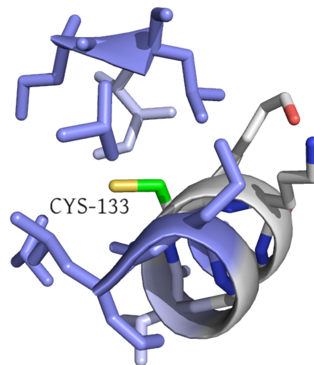
2BUJ:A
