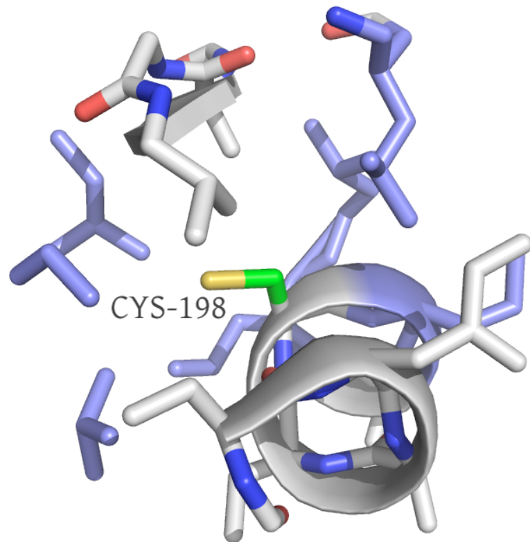
2AVD:A
