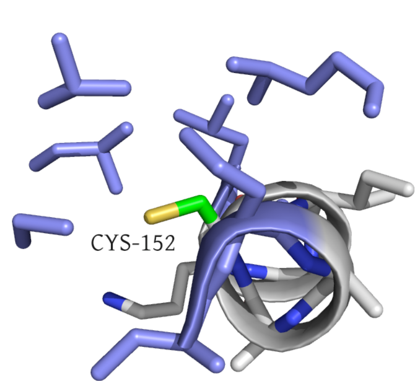
1YQ7:A
