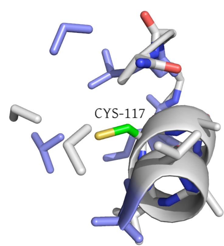
1W66:A
