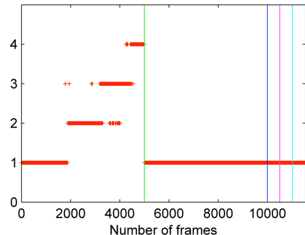
(d) ECL2
