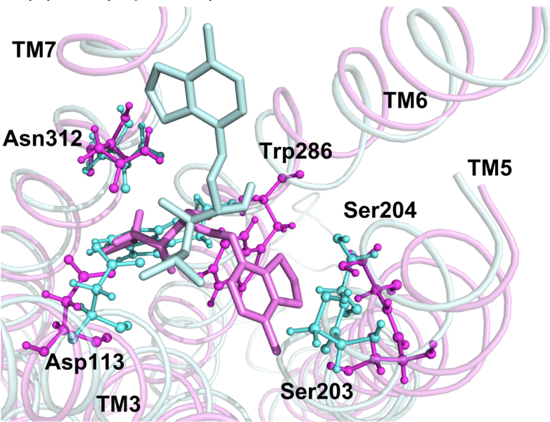
(c) ICI (top view)
