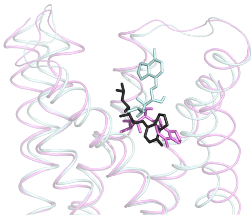
(d) ICI (side view)
