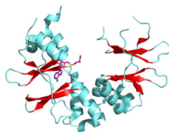
2YZQ_5671432_10_98_11_12
