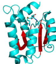
3Q7E_54123
