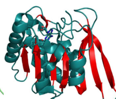
1JG1_7654123
