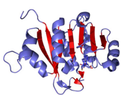
3GRR_3214576
