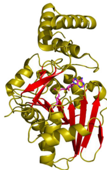
2E58_3421567
