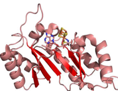
3RFA_654321
