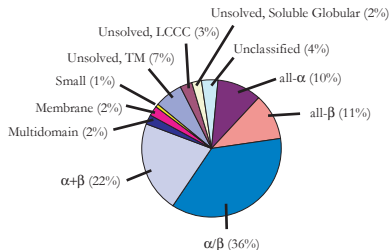
Blochmannia floridanus
