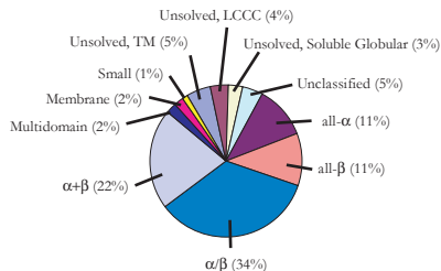
Buchnera aphidicola
