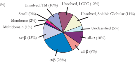
Escherichia coli
