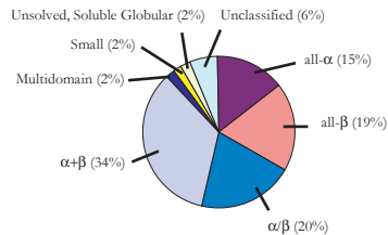
Escherichia coli
