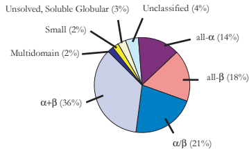
Blochmannia floridanus
