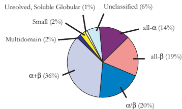
Buchnera aphidicola
