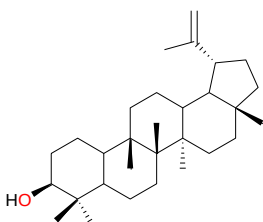
lupeol (11)
