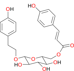
eutigoside A (5)
