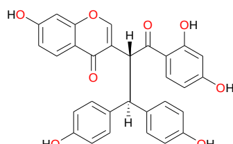
lophirone A (18)
