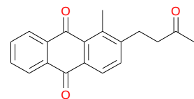
sterequinone F (1)
