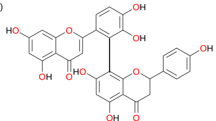
amentoflavone (16)
