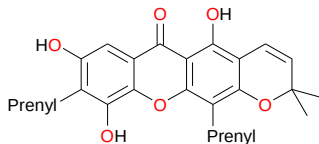
laurentixanthone C (6)
