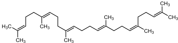
Squalene
