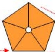
Pentamer
