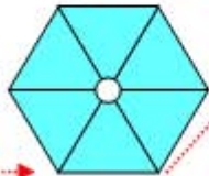
Hexamer
