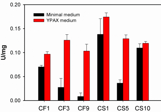
XDH
