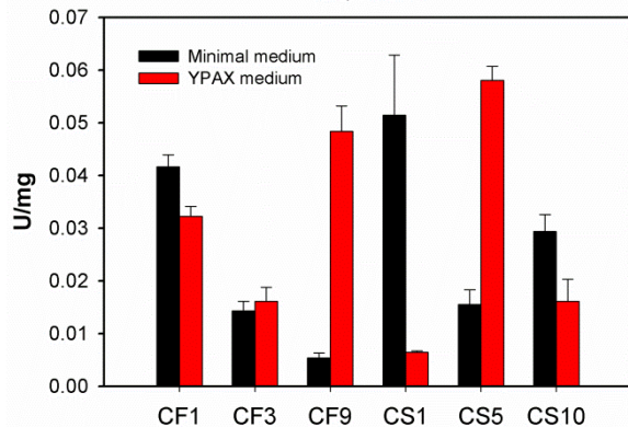
XR, NADH
