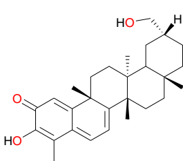
Isoiguesterinol ( 102 )
