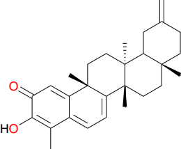
Isoiguesterin ( 100 )
