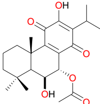
7 \alpha -Acetoxy-6,12-dihydroxy-abieta- 8,12-Diene-11,14-dione ( 112 )
