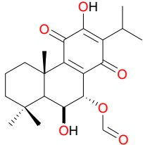
7 \alpha -Formyloxy-6,12-dihydroxy-abieta- 8,12-Diene-11,14-dione ( 111 )
