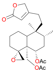
Ajugarin-1 (126)
