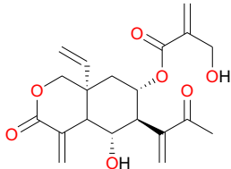
Vernodalol (122)
