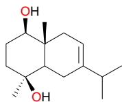
Oplodiol (129)
