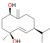
5E,10(14)-germacradien-1 \beta ,4 \beta -diol (128)
