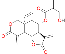
Vernodalin (121)
