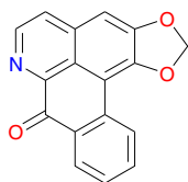
Liriodenine (13)
