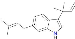
Caulidine A (8)
