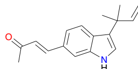
Caulidine B (9)
